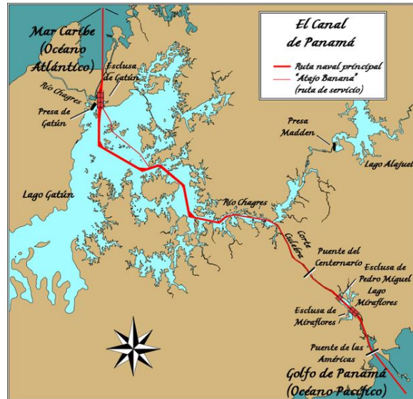
FIGURA 9 DIAGRAMA DEL CANAL DE PANAMÁ
